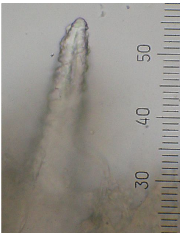
シスチジア(水封入)
